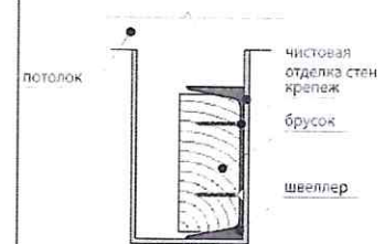
Конструкция внутри проема
