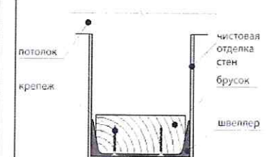
Конструкция внутри проема
